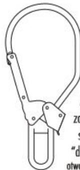
AZ 023 zatrzaśnik duraluminiowy "duży hak" otwarcie 64 mm
